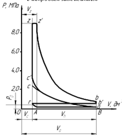
Рис. 4.2. Индикаторная диаграмма четырехтактного дизельного двигателя
