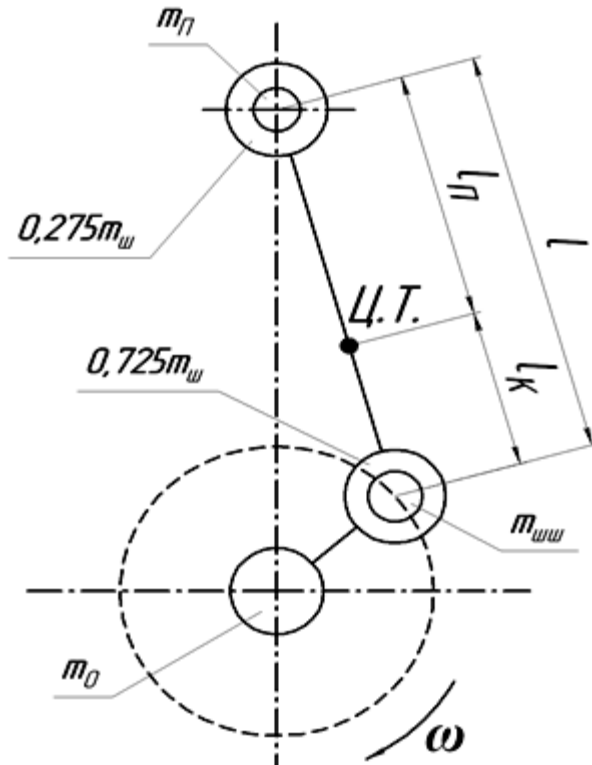
Рис. 4.4. Схема приведения масс КШМ
