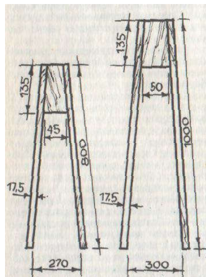
Рис. 12. Правилки для шкурок
