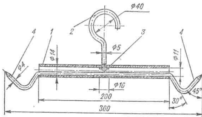
Рис. 8. Вешалка-распорка
