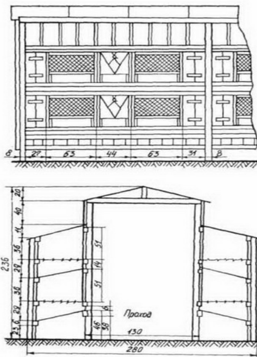
Рис. 16. Схема двухъярусного шеста для кроликов
