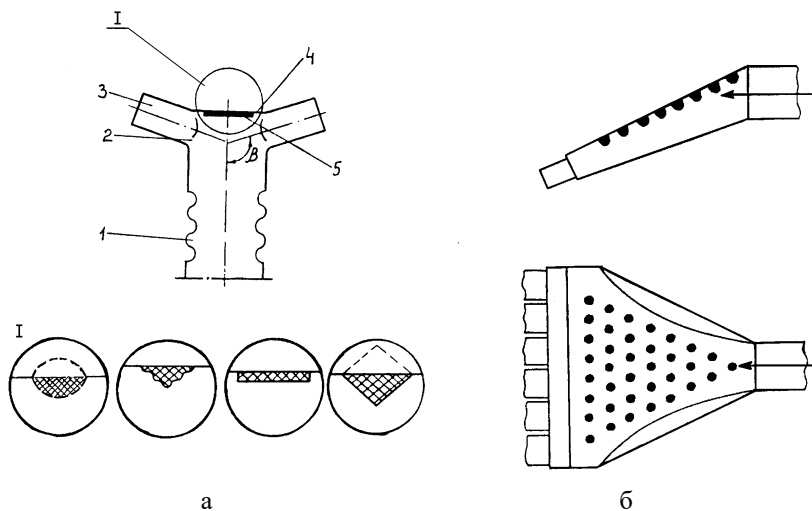
Рис. 3.13. Схемы распределительных головок высевальных систем: а – цилиндрической: 1 – направляющий; 2 – коллектор; 3 – выходные патрубки; 4 – крышка; 5 – отражатель; б – плоской
