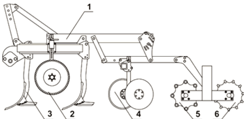
Рис. 19. Культиватор Smaragt
