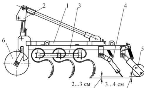
Рис. 28. Культиватор блочно-модульный КБМ-4,2НУ (вид слева): 1 – рама несущая; 2 – навесное устройство; 3 – сменный модуль; 4 – планоно-зубовой выравниватель; 5 – борона роторная (каток); 6 – колесо опорное
