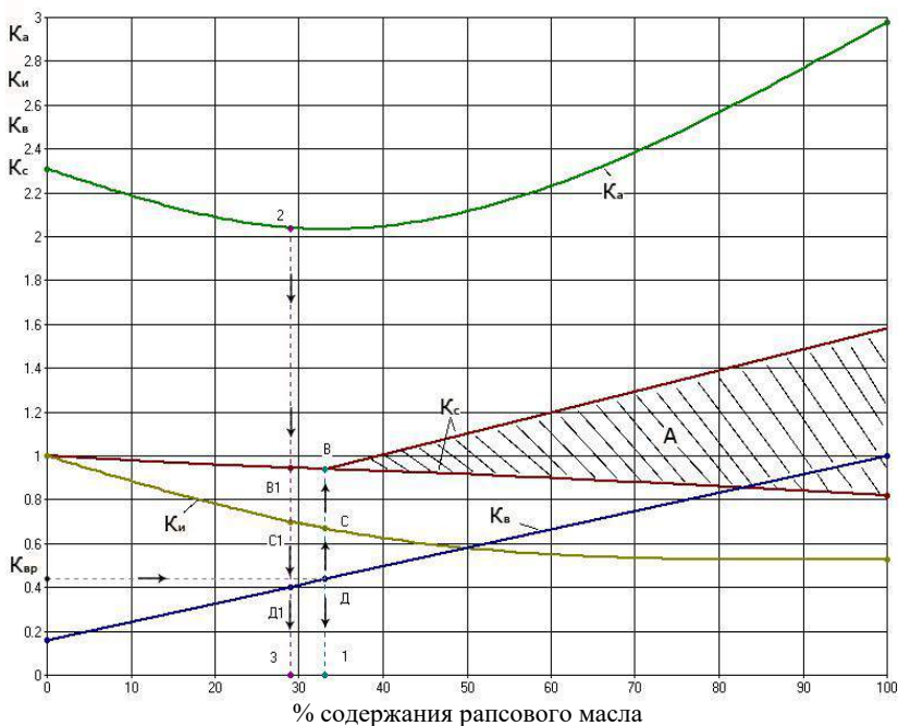
Рис. 11.8. Изменение критериев оптимизации состава смеси минерально-растительного топлива
