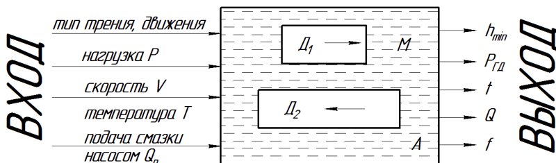
Рис. 15.2. Элементарная трибологическая система ДВС: h_{min} – минимальная толщина масляного слоя; P_{гд} – гидродинамическое давление масла в слое; t – температура масла в подшипнике; Q – расход смазки через подшипник; f – коэффициент трения
