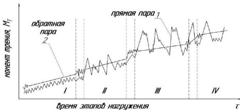
Рис. 9.3. Колебания момента трения
