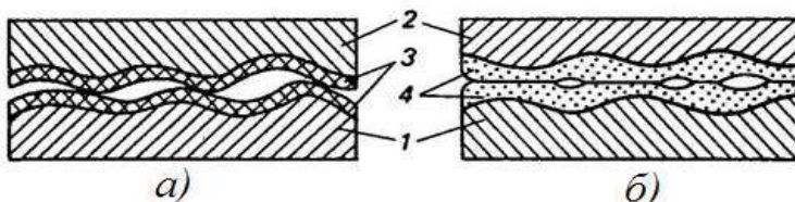
Рис. 8.4. Поверхности контакта деталей: а – при граничной смазке; б – при ИП; 1 – сталь; 2 – бронза; 3 – окисные пленки; 4 – сервовитные пленки
