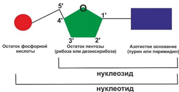
Рис. 1.1. Строение нуклеотида и нуклеозида
