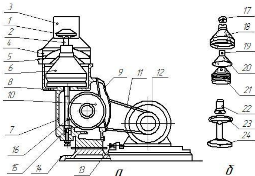
Рис. 4. Сепаратор СМ-3-1000М:
