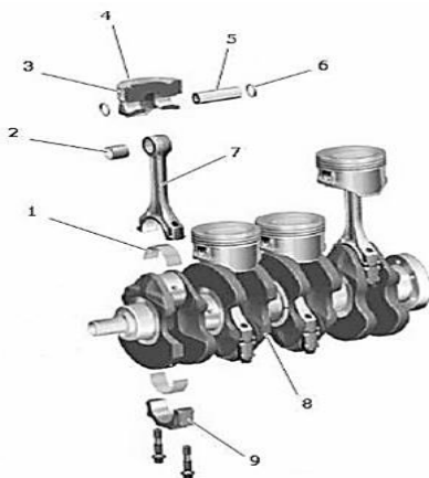
Рис. 9. Схема КШМ:
