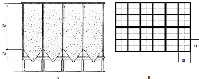
Рис. 4. Силос прямоугольного сечения: А) внешний вид, профиль: H – высота прямоугольной части силоса, H_1 – высота трапецевидной части силоса. Б) внешний вид сверху: \text{Ш} – ширина силоса квадратного сечения, D – длина силоса квадратного сечения
