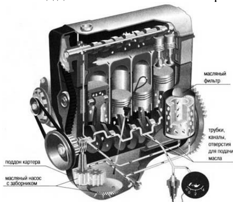
Рис. 10. Система смазки двигателя:
