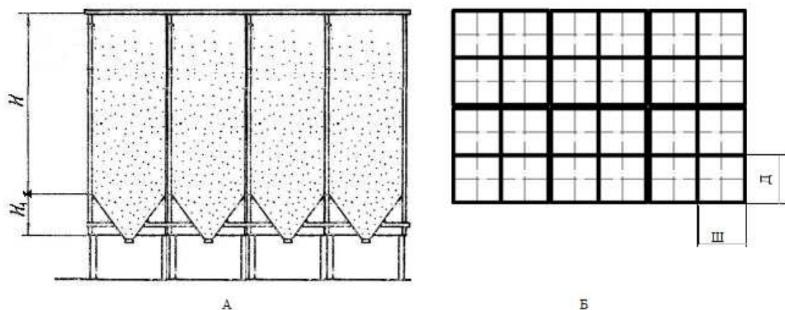
Рис. 4. Силос прямоугольного сечения: А) внешний вид, профиль: H – высота прямоугольной части силоса, H_1 – высота трапецевидной части силоса. Б) внешний вид с верху: \Pi – ширина силоса квадратного сечения, D – длинна силоса квадратного сечения
