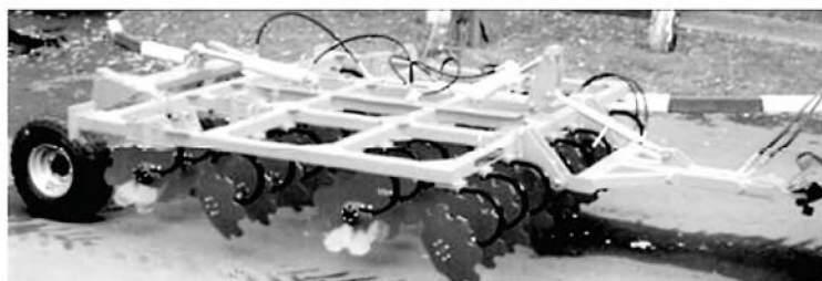
Рис. 32. Дисковый мульчировщик ДМ-3,2
