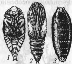
Рис. 1.26. Типы куколок: 1 — открытая; 2 — покрытая; 3 — скрытая
