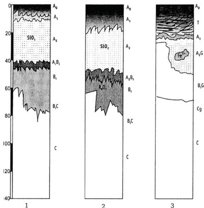
Рис. 7. Строение почв таежно-лесной зоны:
