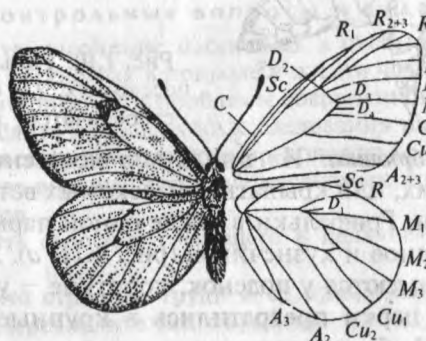
Рис. 1.9. Жилкование крыльев бабочки-боярышницы: C — ко- стальная жилка; Sc — субко- стальная; D 2-4 — дискальные жилки; R 1 , R 2+3 , R 4 , R 5 — радиальные жилки; M 1-3 — медиальные жилки; Cu 1-2 — кубитальные жилки; A 2 , A 2+3 , A 3 — анальные жилки
