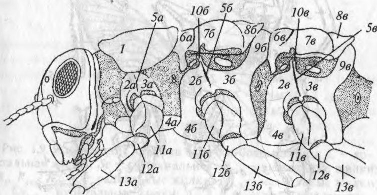
Рис. 1.7. Схема строения и подразделения на склериты груди насекомого (по Шванвичу): 1 — переднеспинка; 2 — эпистерн передне-, средне- или заднегрудь; 3 — их эпимеры; 4 — их грудка; 5 — их плеиральный шов; 6 — предшит средне- и заднеспинки; 7 — их шит; 8 — их щитик; 9 — их заспинка; 10 — плеиральный столбик; 11 — тазик передних, средних и задних ног; 12 — их вертлуг; 13 — их бедро; индексы a , б , в обозначают принадлежность к передне-, средне- или заднегрудь
