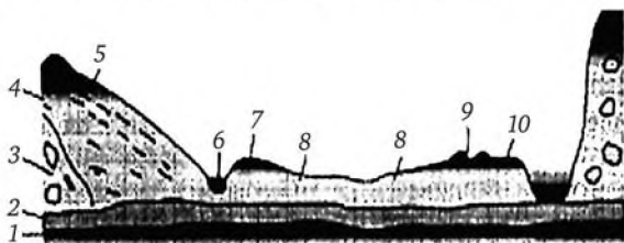
Рис. 11. Поперечный разрез через долину реки:
