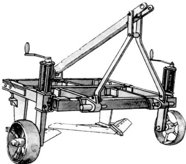
Рис. 18. Плоскорез-глубокорыхлитель КПГ-2-150
