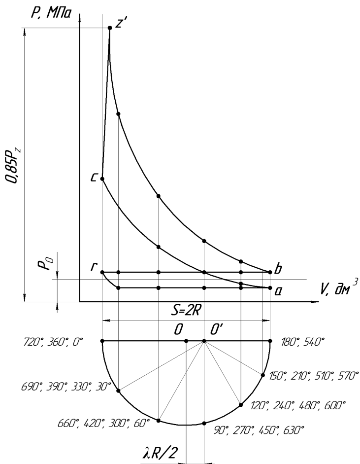
Рис. 4.4. Индикаторная диаграмма с поправкой Ф.А. Брикса
