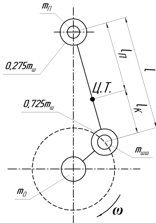
Рис. 4.2. Схема приведения масс КШИМ
