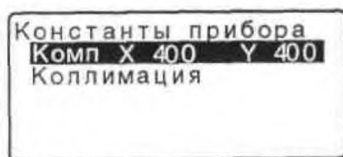
Рис. 16. Проверка компенсатора наклона вертикальной оси
