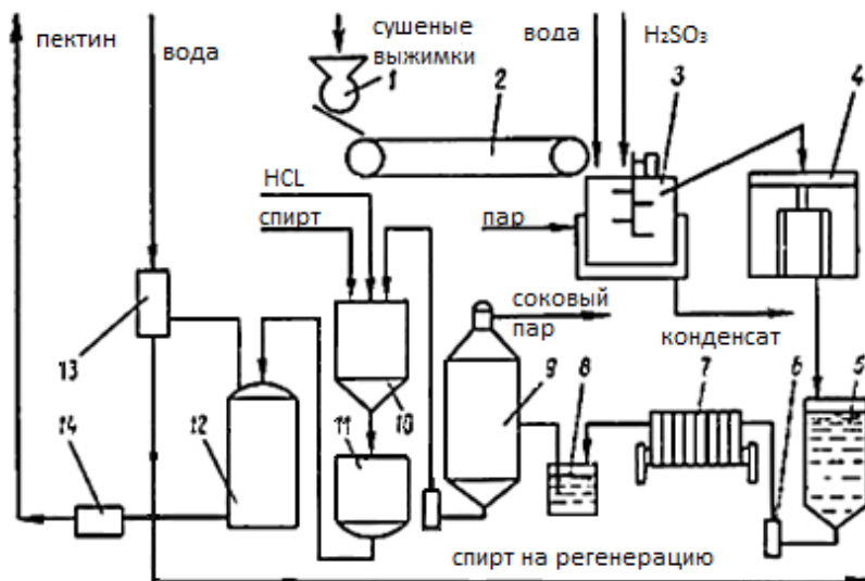
Рис. 8. Технологическая схема получения пектина из яблочных выжимок:
