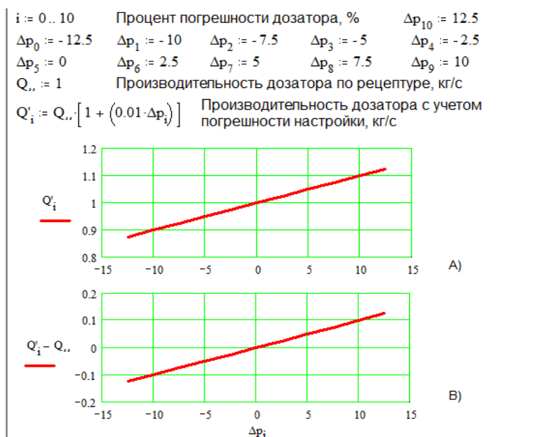
Рис. 2. Листинг текстовой части программы в математическом пакете MatchCAD по определению влияния погрешности настройки конкретного дозатора \Delta p_i (%) на: А) заданную производительность его дозатора Q_i , кг/с; В) фактическое отклонение значений производительности дозатора ( Q_i - Q ), кг/с
