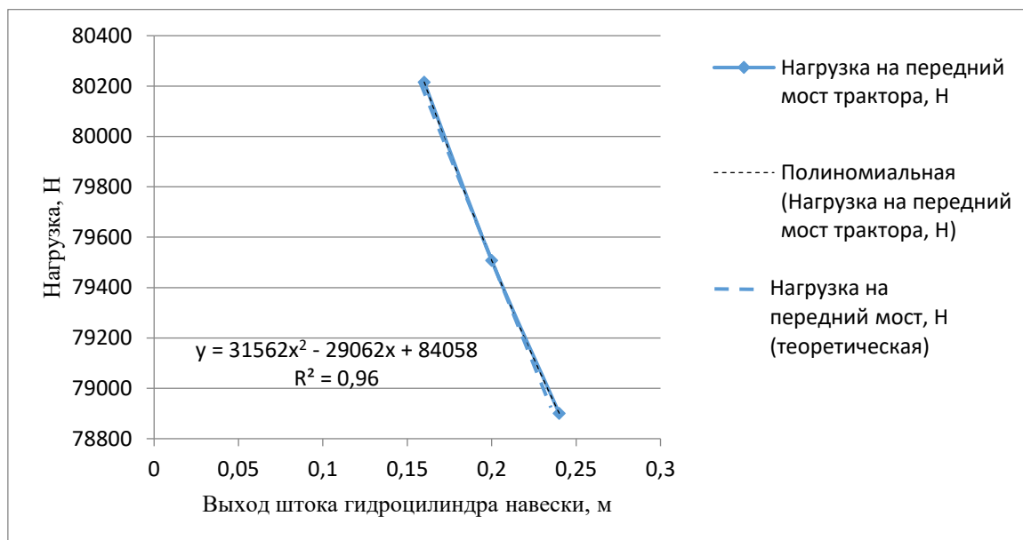
Рис. 2. Зависимость нагрузки на передний мост трактора от выхода штока гидроцилиндра навески (при передаче нагрузки с бороны на трактор)
