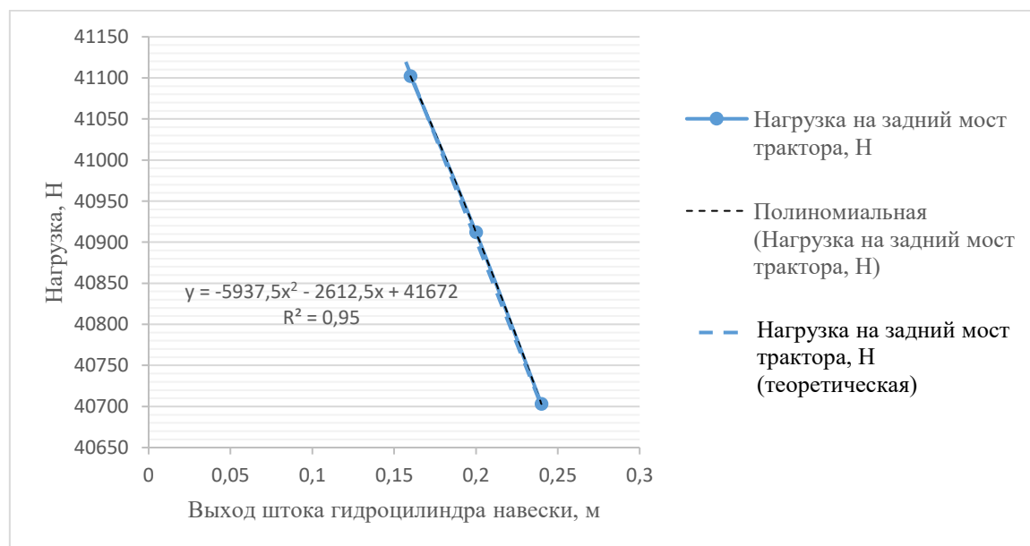
Рис. 3. Зависимость нагрузки на задний мост трактора от выхода штока гидроцилиндра (при передаче нагрузки с бороны на трактор)
