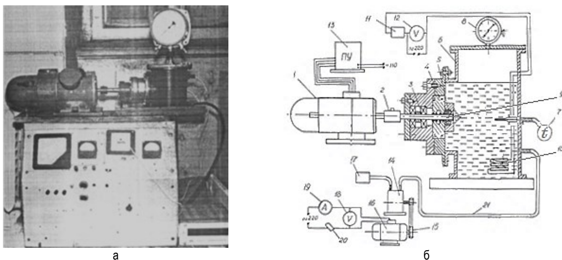
Рис. 1. Экспериментальный стенд для определения герметичности уплотнений:
