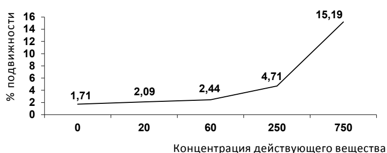
Рис. 1. Зависимость подвижности меди от концентрации действующего вещества, %
