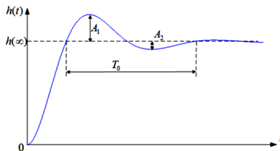
Рис. 2. Графическое определение параметров T колебательного объекта 2-го порядка
