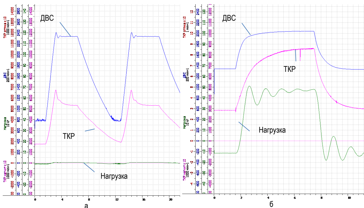
Рис. 4. Динамические характеристики турбокомпрессора и двигателя Д-245-35 (утечка газов перед турбиной, через отверстие диаметром 12 мм): а – без нагрузки; б – под нагрузкой
