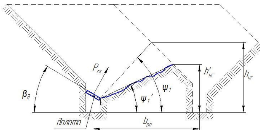
Рис. 3. К определению высоты гребней в зависимости от угла постановки рабочей поверхности долота в поперечно-вертикальной плоскости \beta_o
