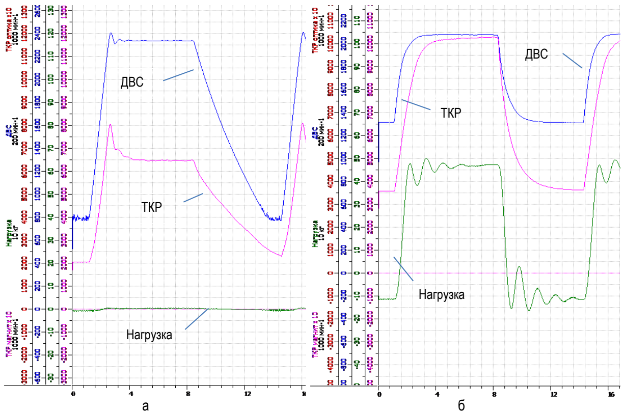
Рис. 5. Динамические характеристики турбокомпрессора и двигателя Д-245-35 (утечка газов после компрессора, площадь отверстия 20 мм 2 ): а – без нагрузки; б – под нагрузкой
