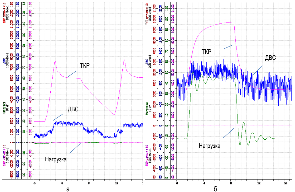
Рис. 6. Динамические характеристики турбокомпрессора и двигателя Д-245-35 (засорение воздушного фильтра, 0,1 МПа): а – без нагрузки; б – под нагрузкой
