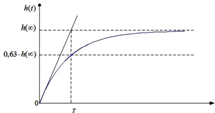
Рис. 3. Графическое определение постоянной времени T инерционного объекта 1-го порядка
