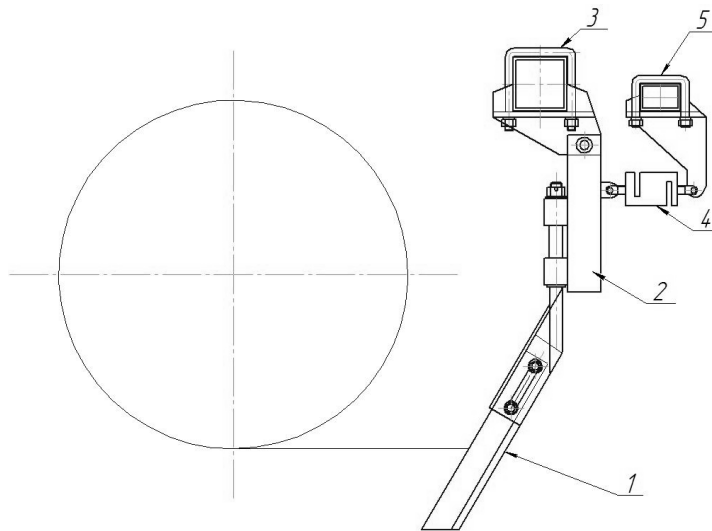
Рис. 1. Конструктивная схема устройства для измерения тягового сопротивления
