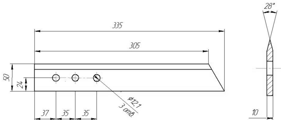
Рис. 2. Деформатор
