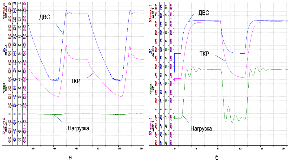
Рис. 1. Динамические характеристики турбокомпрессора и двигателя Д-245-35 (исправное состояние системы): а – без нагрузки; б – под нагрузкой
