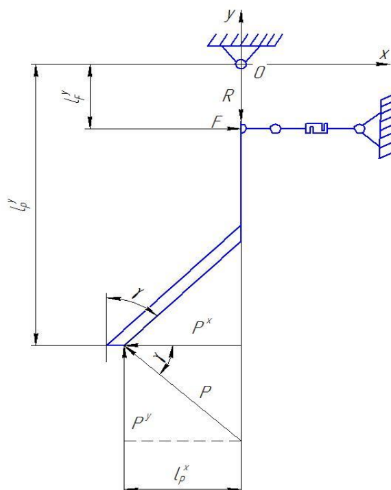
Рис. 3. Схема сил, действующих на тензометрический узел
