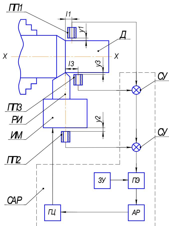
Рис. 1. Схема системы активного контроля и автоматического регулирования размеров детали
