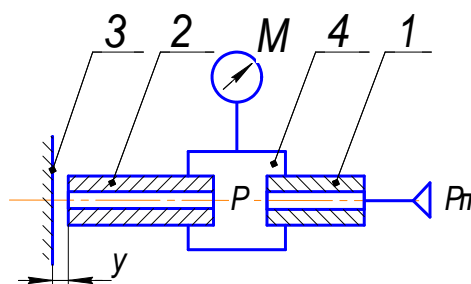
Рис. 2. Полумостовая схема пневматического измерительного преобразователя: 1 – подводящая трубка пневмоподачи; 2 – сопло пневмоподачи; 3 – деталь; 4 – регулятор давления; М – манометр
