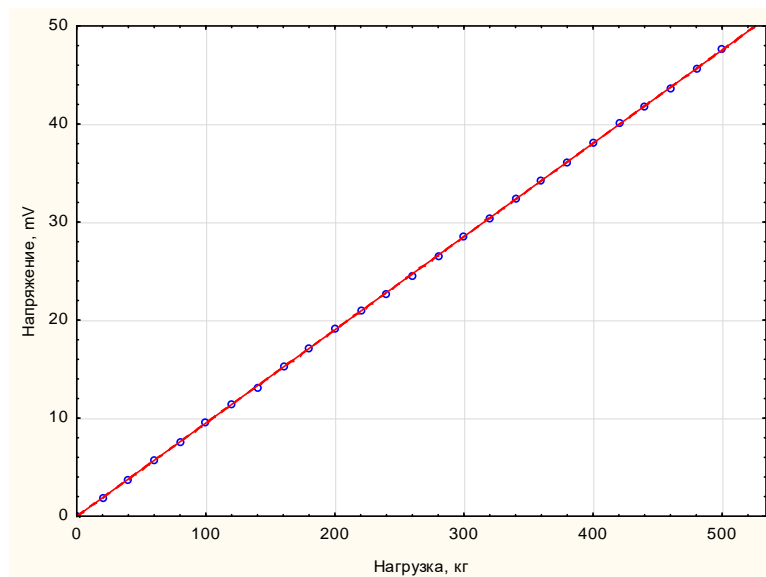
Рис. 3. Усреднённый тарировочный график 8 датчиков С2Н, доверительный интервал 95%
