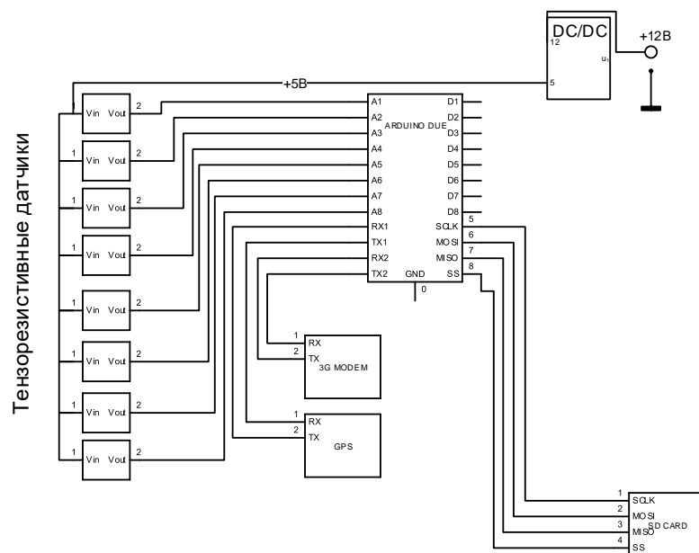
Рис. 2. Электрическая схема экспериментальной системы
