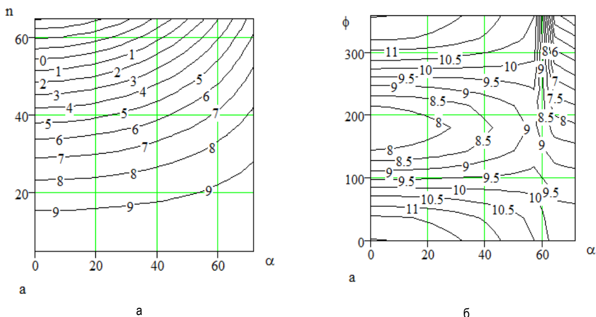
Рис. 5. Влияние конструктивных параметров на величину вертикальной проекции ускорения a_v ( \text{m}/\text{c}^2 ): а – угла наклона барабана \alpha (град.) и частоты вращения барабана n ( \text{мин}^{-1} ) при D=0,6 м и \varphi=180^\circ ; б – угла наклона барабана \alpha (град.) и угла расположения частиц \varphi (град.) при D=0,6 м и частоте вращения барабана n=26 \text{мин}^{-1}
