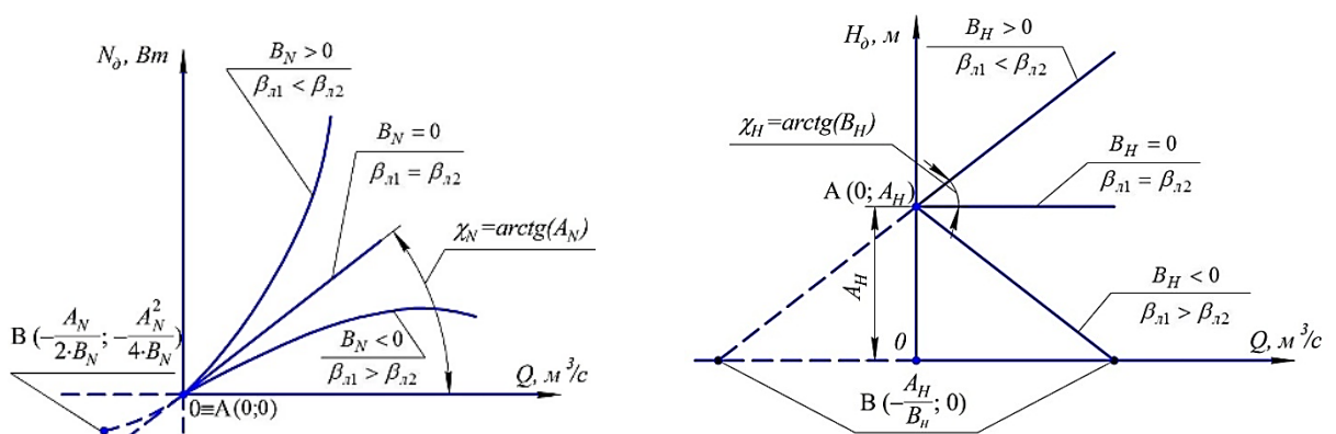
Рис. 2. Схемы к определению графиков зависимости H_{\partial} = f(Q) , N_{\partial} = f(Q) при различных углах \beta_{л1} и \beta_{л2}
